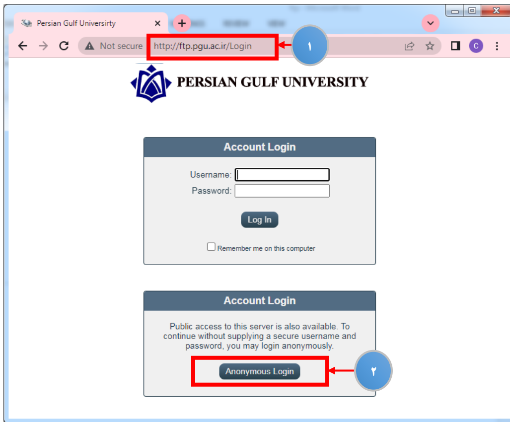
تصویر ۷
